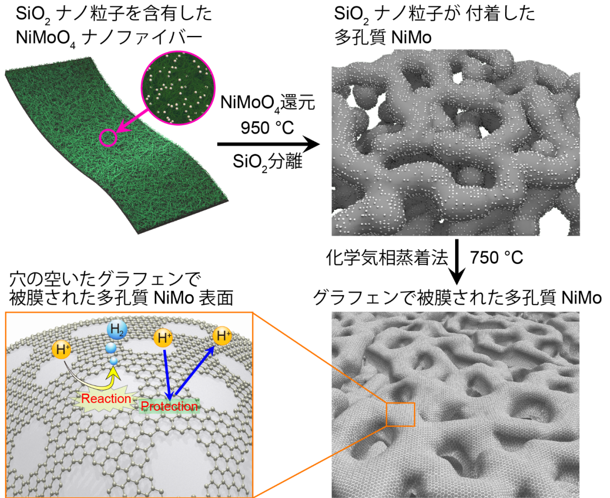
図1 穴の空いたグラフェンで被膜したニッケルモリブデン(NiMo)の作製概要図と水素発生メカニズム。シリカナノ粒子と酸化ニッケルモリブデン(NiMoO 4 )ナノファイバーを混ぜて加熱還元し、連続的に化学気相蒸着法でグラフェンを成長させると、一部穴の開いたグラフェンに覆われているニッケルモリブデン表面が生成する。穴の空いた部分では水素イオン(硫酸水溶液)と表面が接触し水素が発生、穴の空いていない部分では硫酸水溶液との過剰な接触が防がれている。
