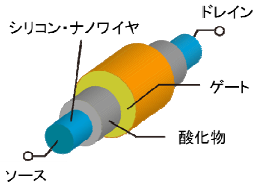
図1 シリコン・ナノワイヤ材を用いた電界効果トランジスタのイメージ
