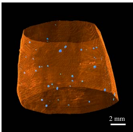
柱状の氷中に分布するエアハイドレート粒
