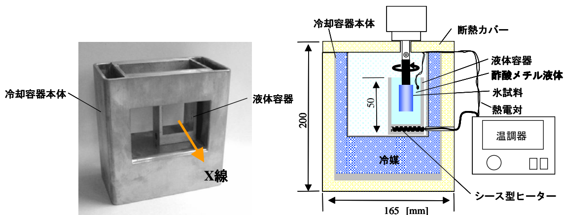
低温試料容器
