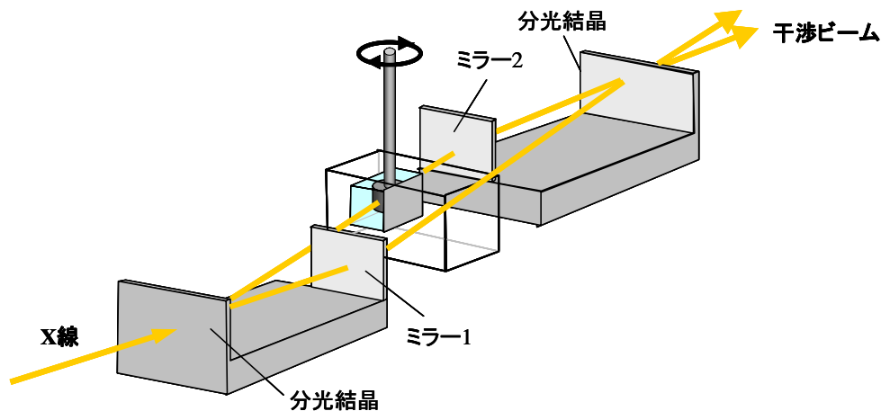
低温型の位相コントラストX線CT測定手法
