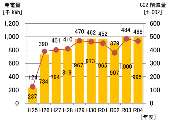
発電量とCO2削減量の推移 (筑波キャンパス太陽光発電設備)
